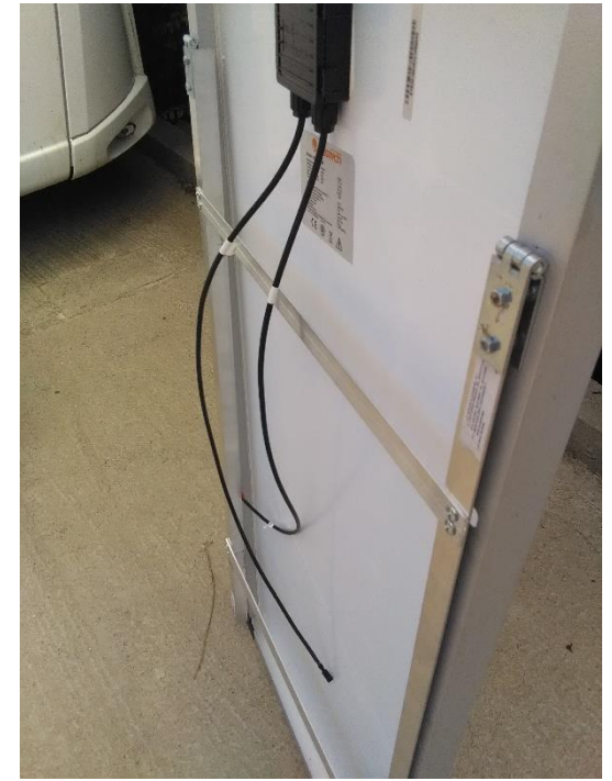
Găurit si montat cu șuruburi de 5 Suportul are deschidere de la 0 la aproape 180° Pliat nu ocupă spațiu în plus
